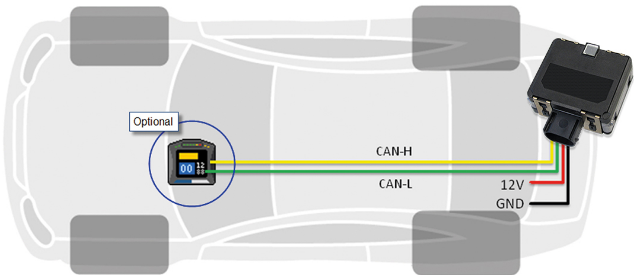
Wiring schematic
