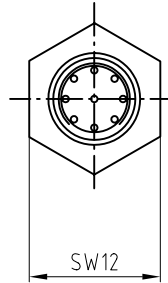
Ansicht A view M 2:1
